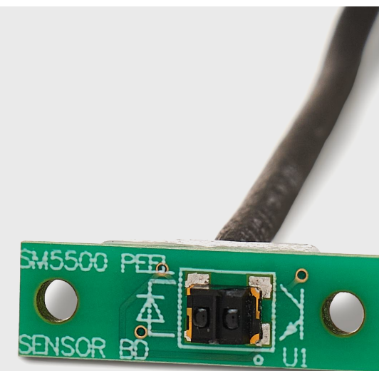
ОПТИЧЕСКИЙ ДАТЧИК С ПРОВОДОМ MOLEX, JST, 1.25MM
